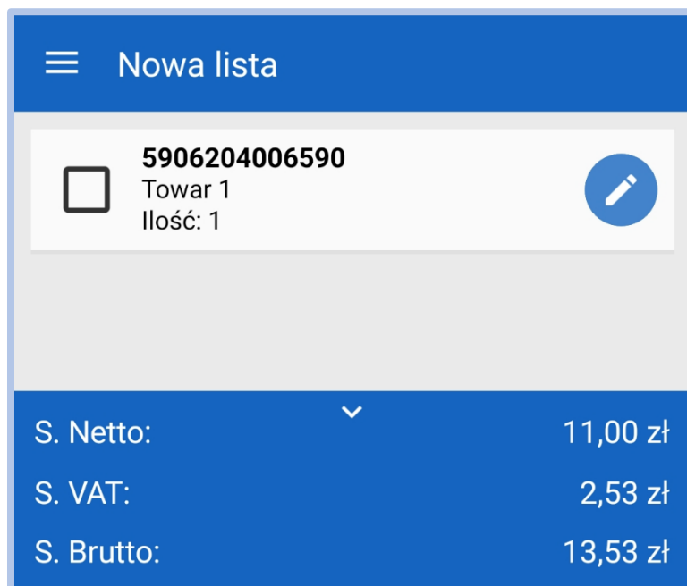
Rys. 11 Podsumowanie
