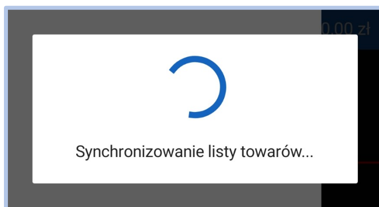
Rys. 8 Okno synchronizacji
