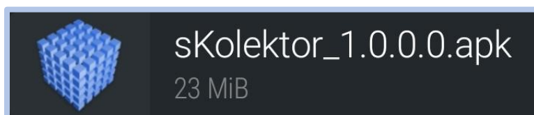
Rys. 1 Plik instalacyjny
