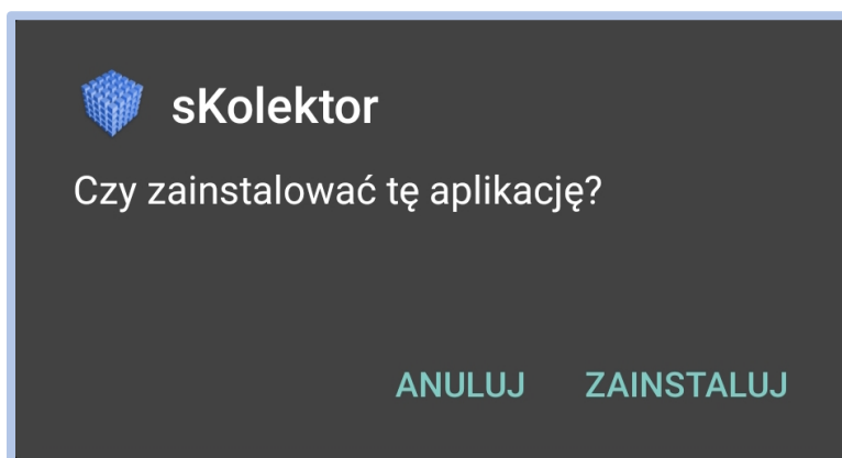
Rys. 2 Okno instalatora
