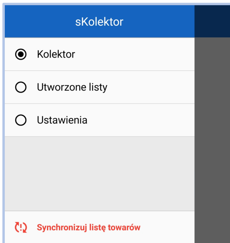
Rys. 5 Menu główne
