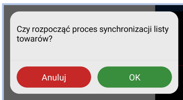
Rys. 7 Okno dialogowe
