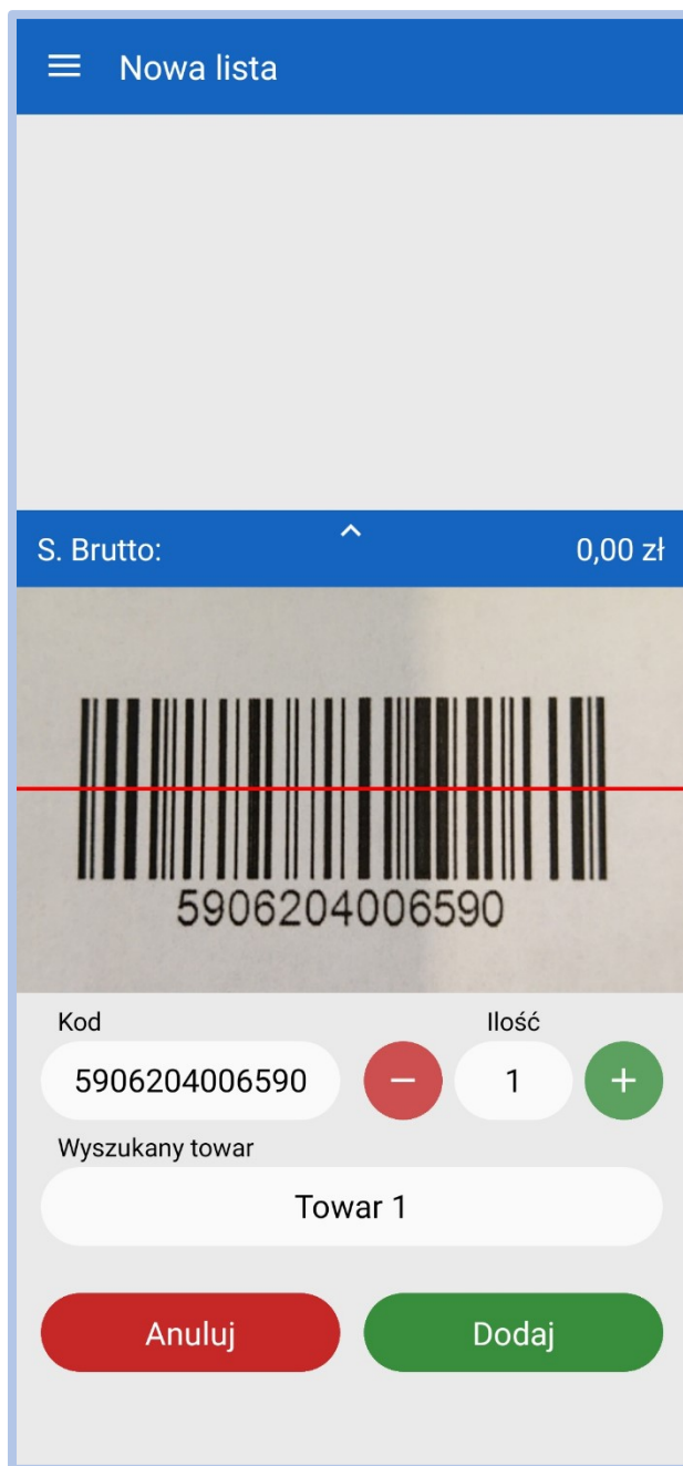
Rys. 10 Okno Kolektor
